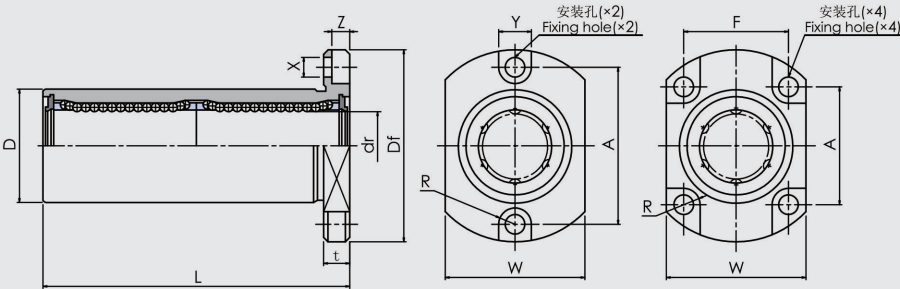
轴径小于或等于12mm LMSH12L or Less 轴径大于或等于16mm LMSH16L or More
